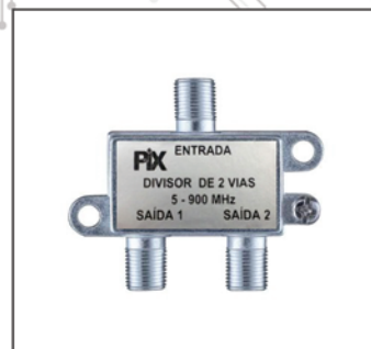
Divisor 2 saídas
